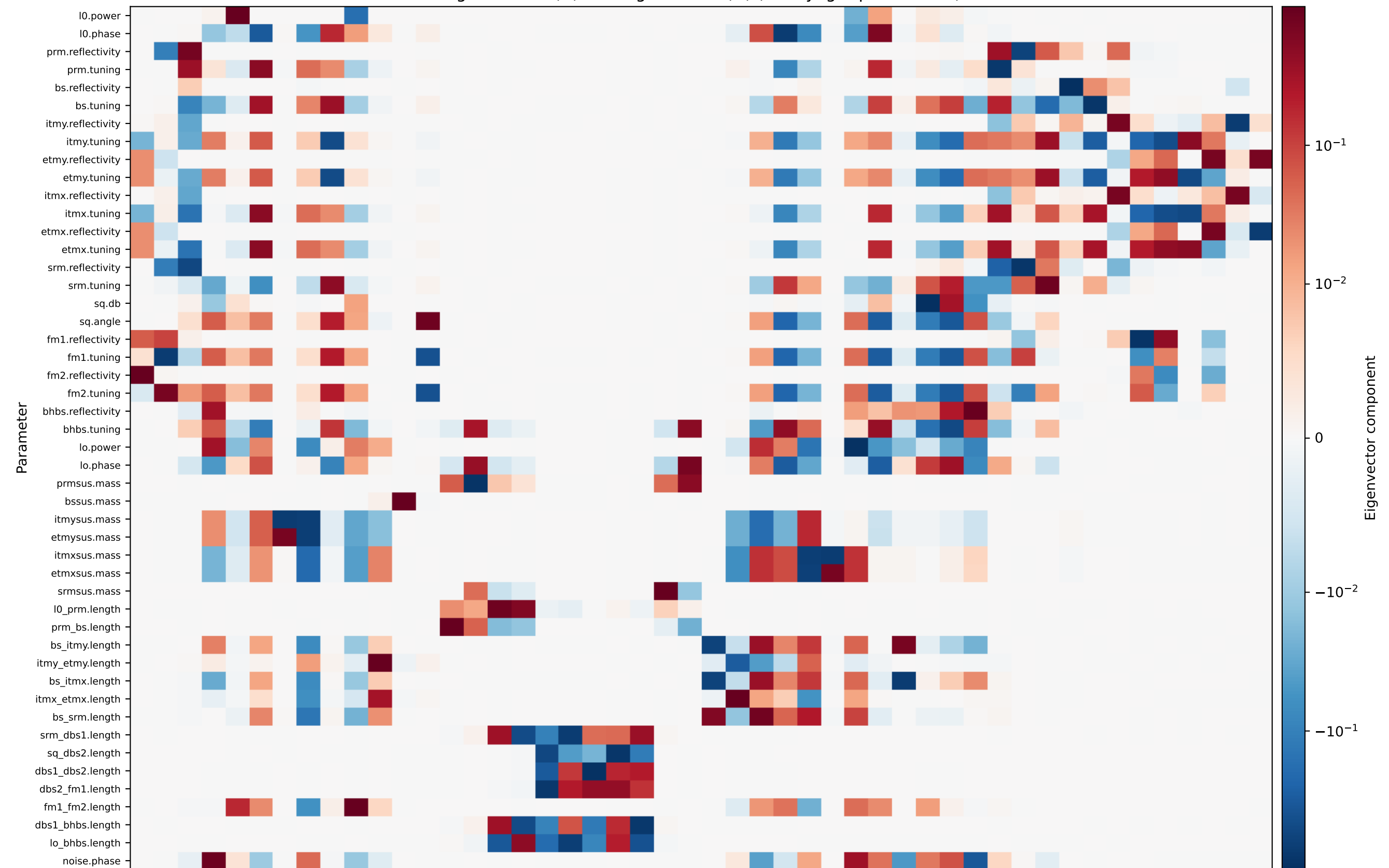
Eigenvectors (U) and eigenvalues (D) (at Voyager parameters)
