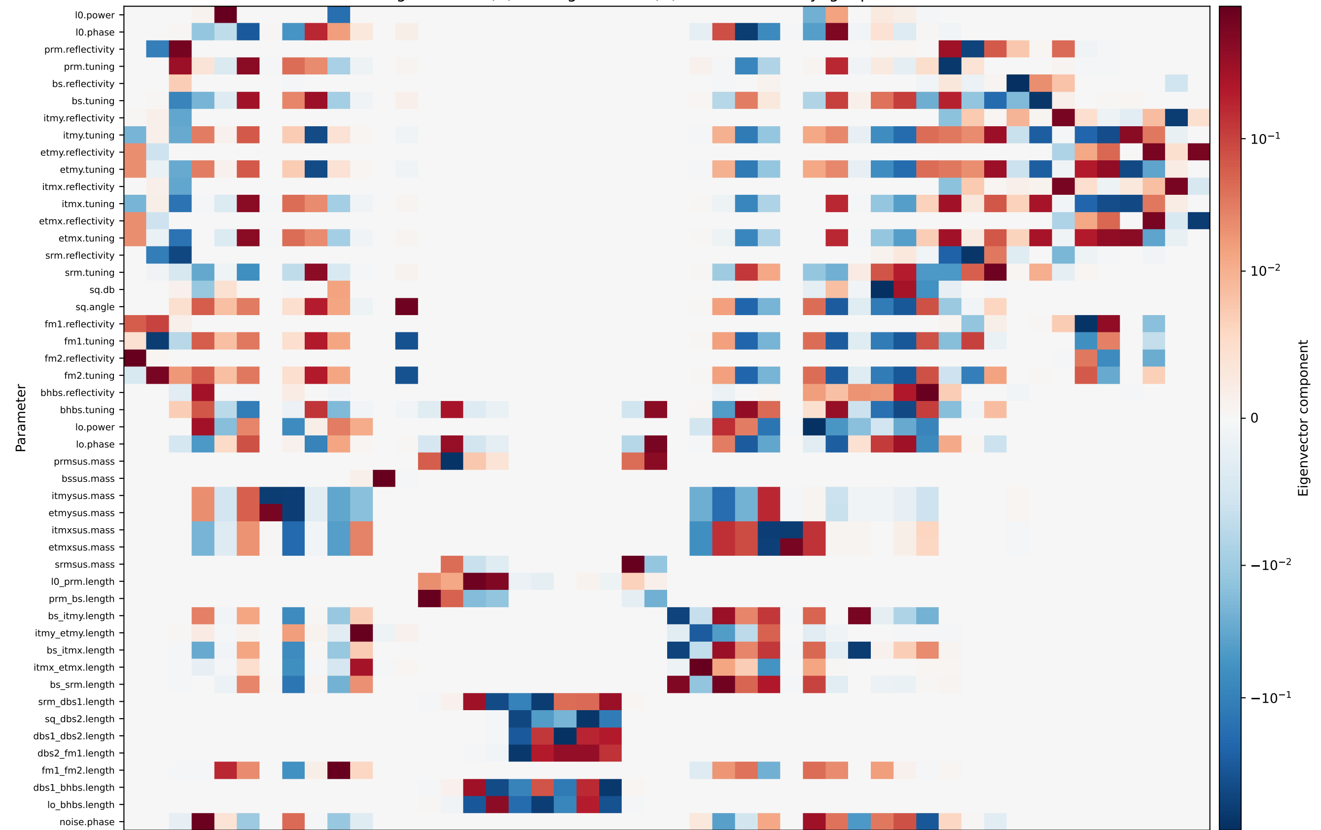
Eigenvectors (U) and eigenvalues (D) of Hessian at Voyager parameters
