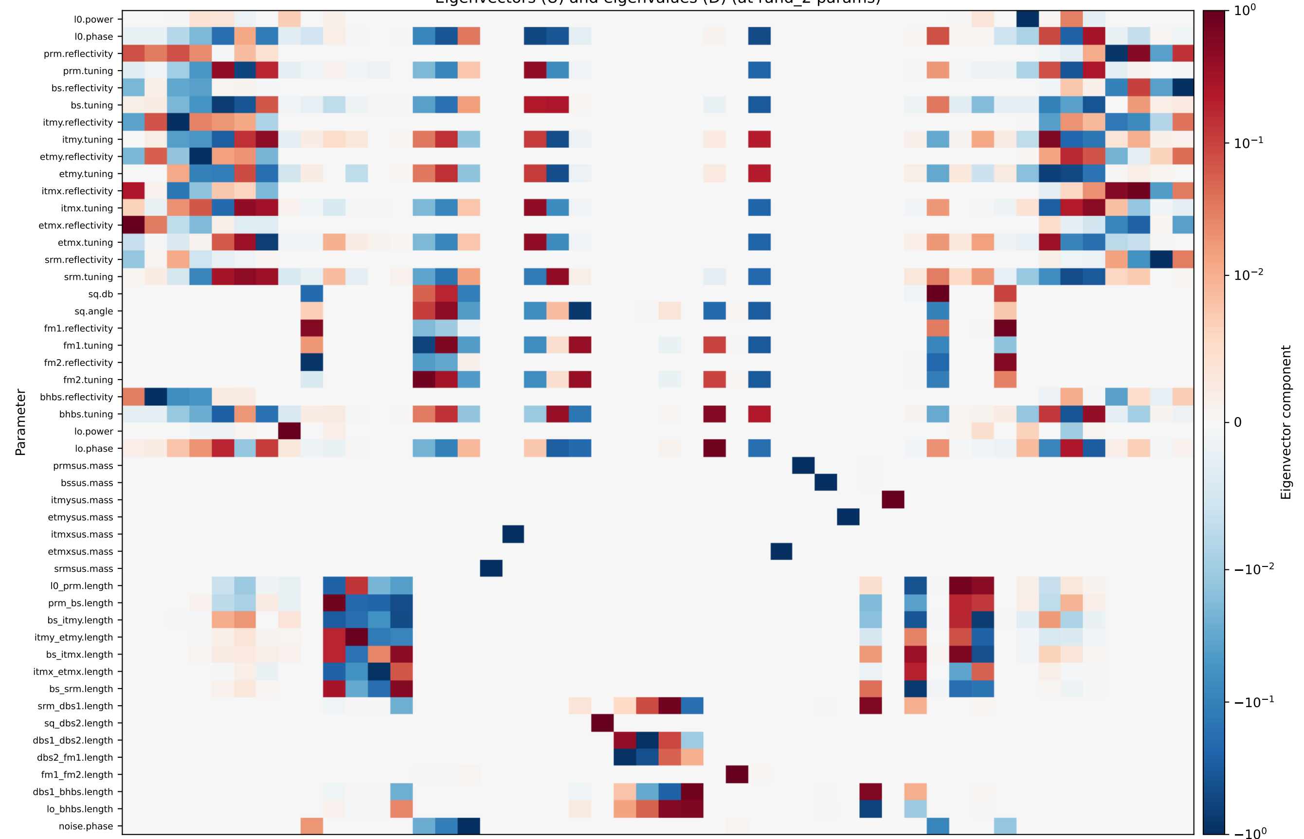
Eigenvectors (U) and eigenvalues (D) (at rand_2 params)
