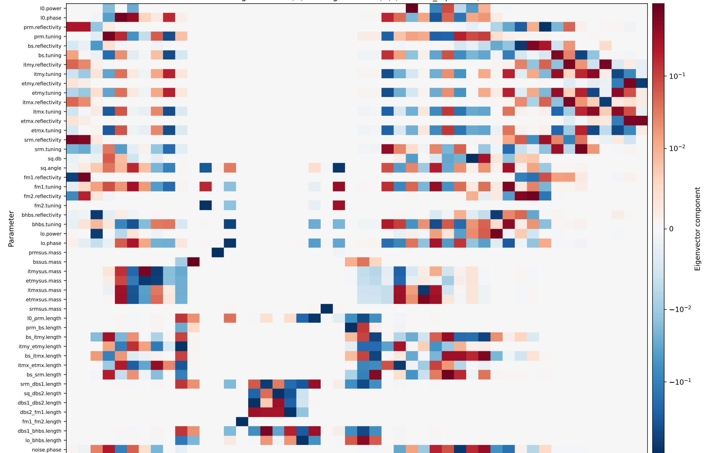
Eigenvectors (U) and eigenvalues (D) (at adam_0 params)
