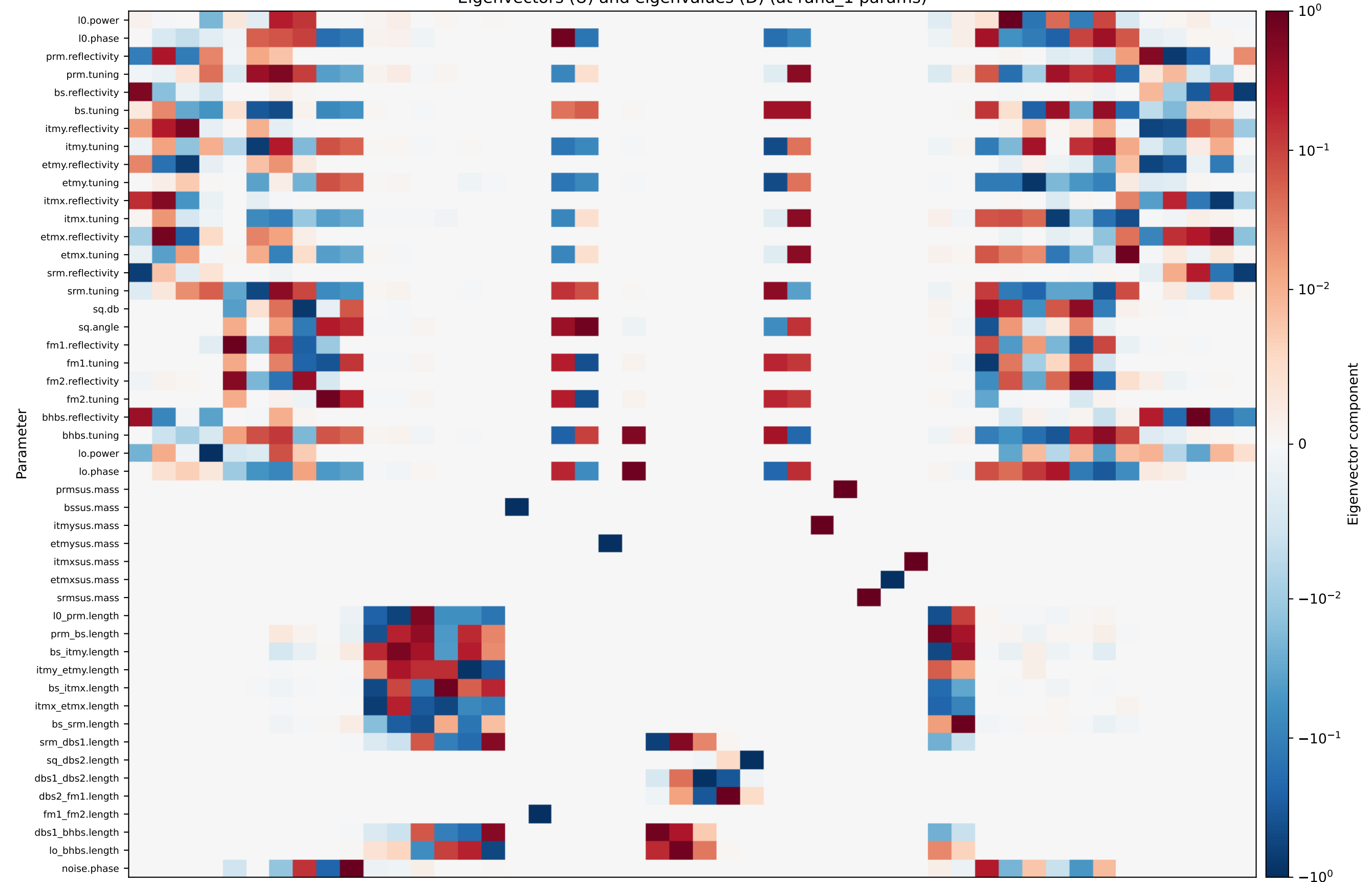
Eigenvectors (U) and eigenvalues (D) (at rand_1 params)
