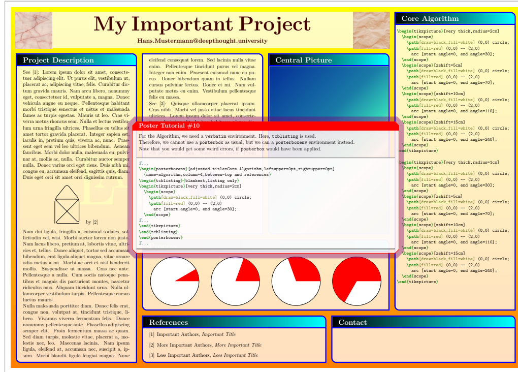
Original tcolorbox
