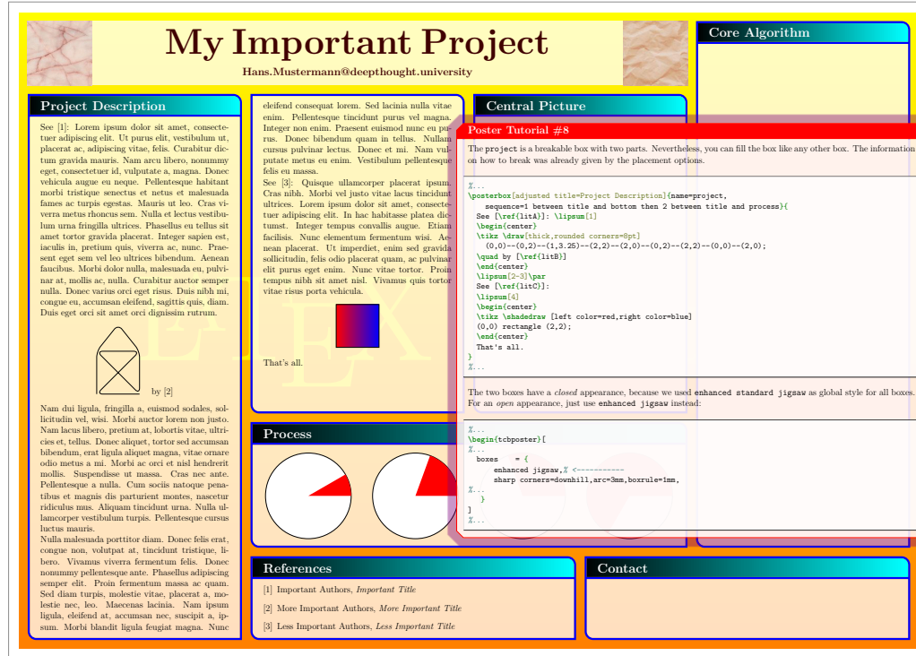
Original tcolorbox
