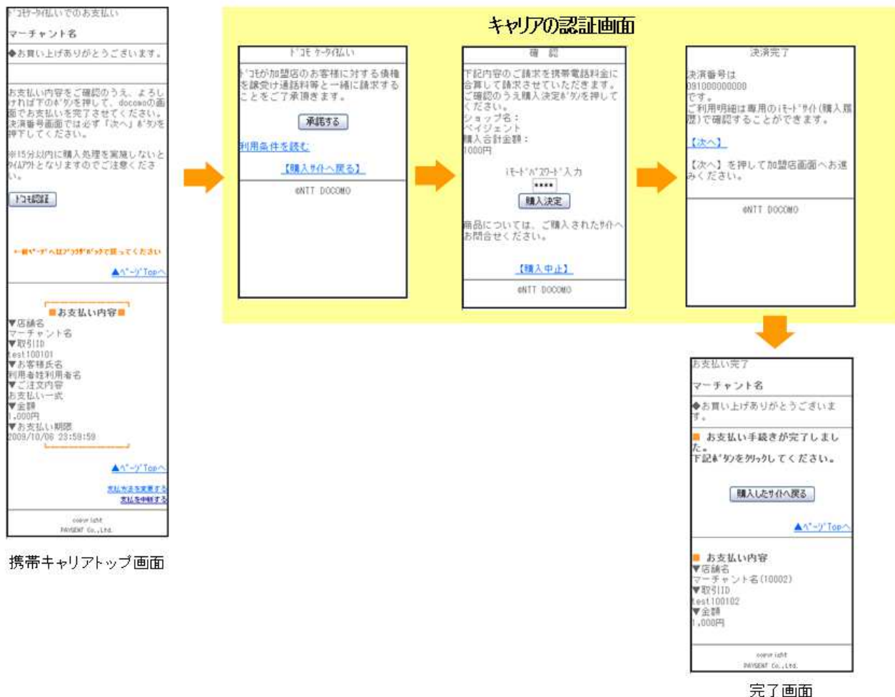
図. 携帯キャリア支払の流れ (d 払いの場合)
