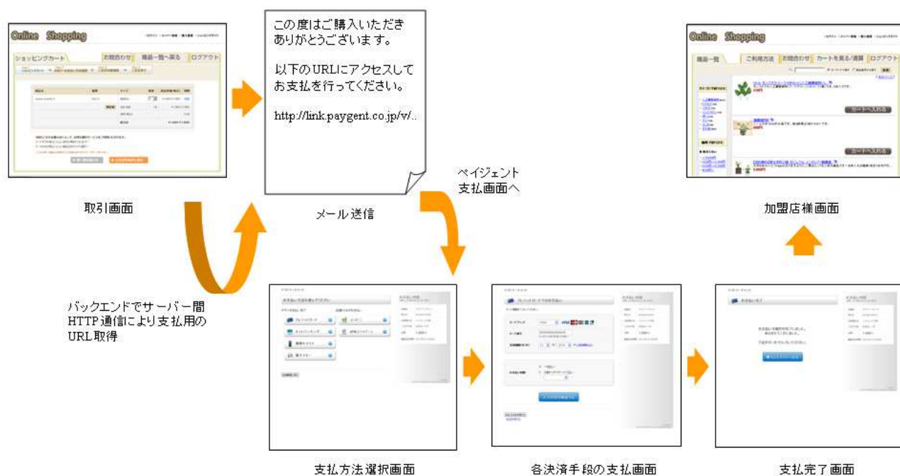
図. URL 連携方式の画面遷移例 - 2
