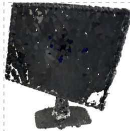
GaussianArt
