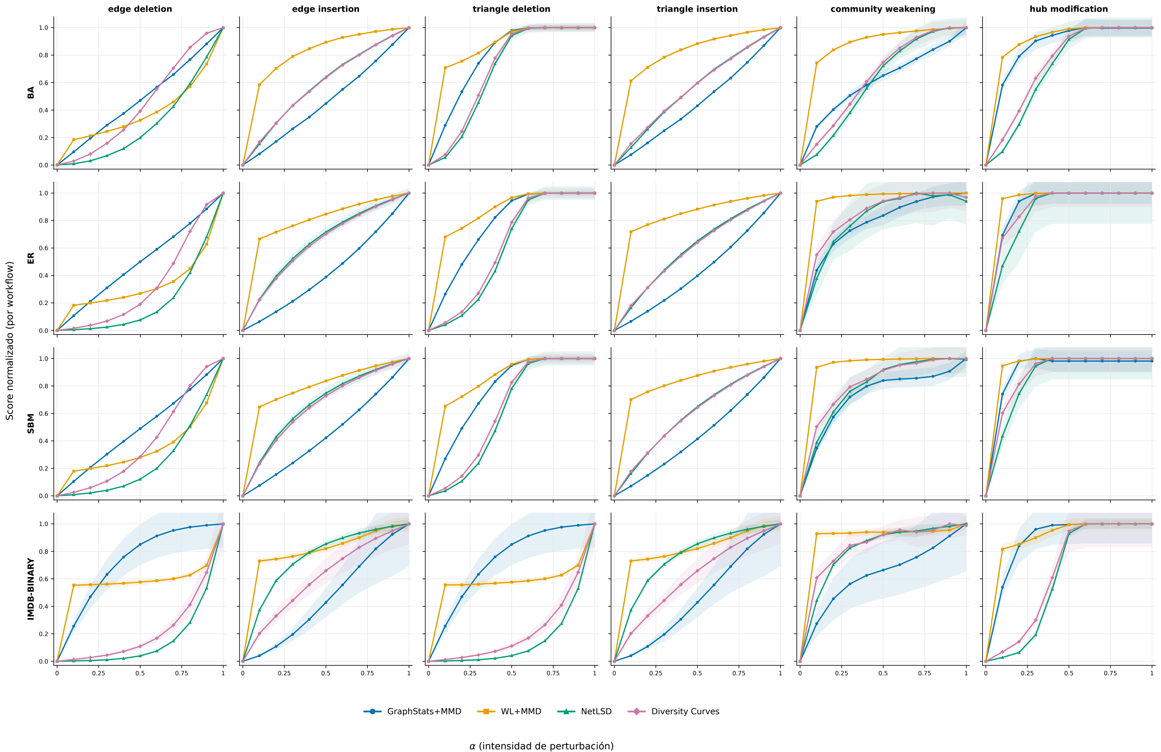
Apendice B. Curvas completas de paired_score vs \alpha (4 datasets \times 6 perturbaciones)
