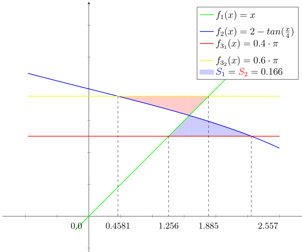
Рис. 4: Плоская фигура, ограниченная графиками заданных уравнений
