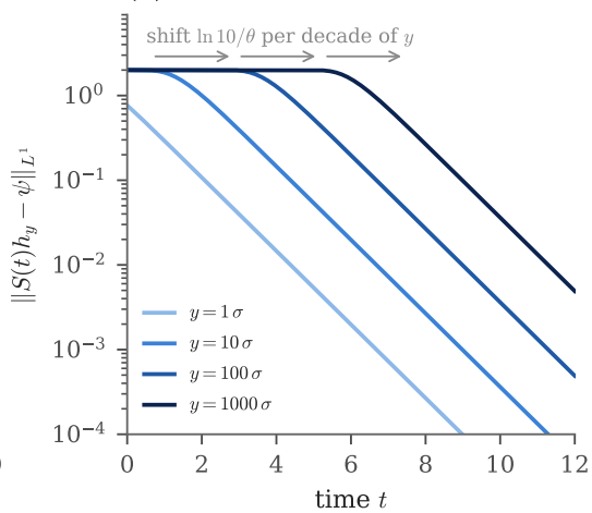
(d) OU: no uniform rate
