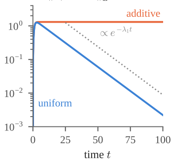
(f) \|u/U - \psi\|_{L^1}
