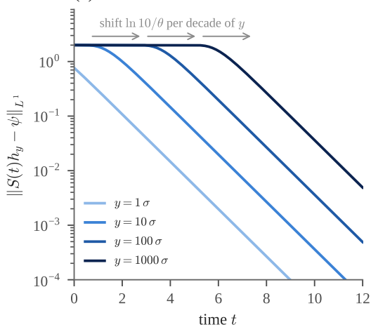
(d) OU: no uniform rate
