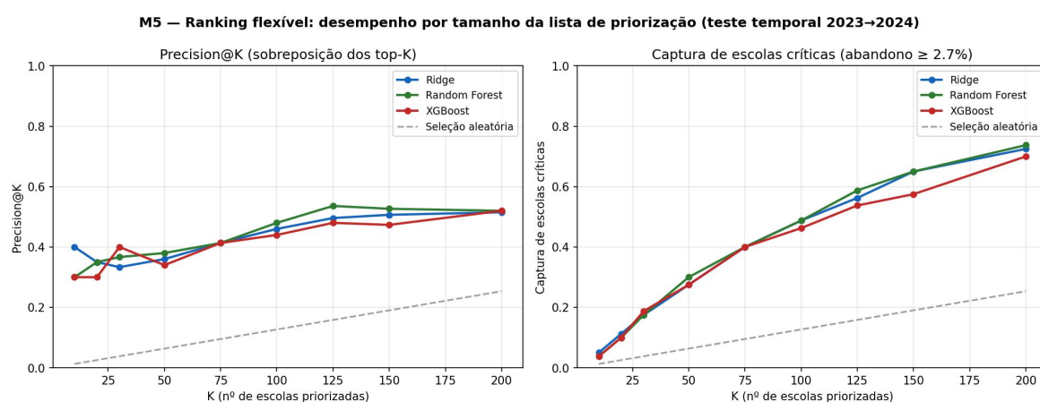
Figura 16 – Acerto e alcance da lista para diferentes tamanhos de lista
