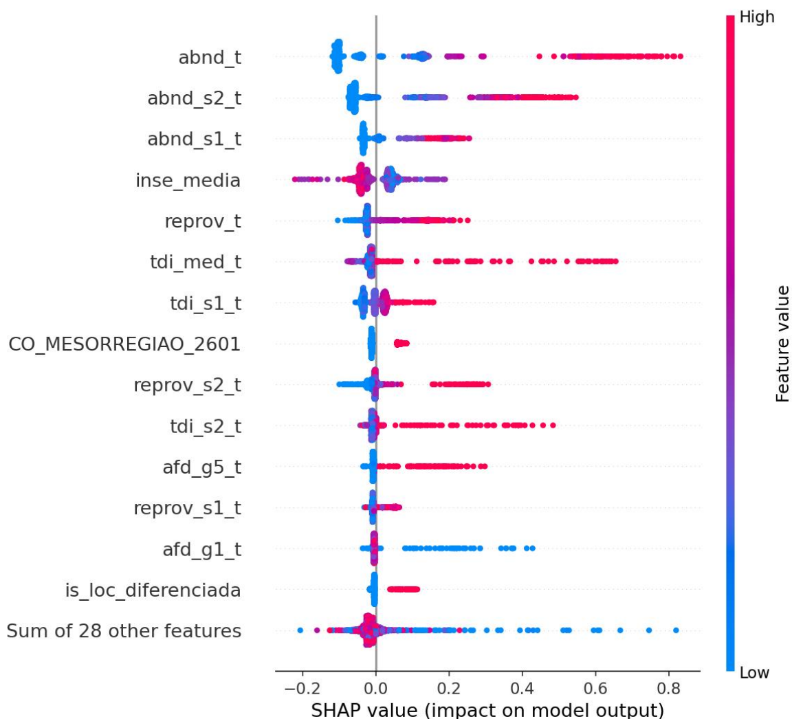
S1 — SHAP global (beeswarm): contribuição por escola e feature
