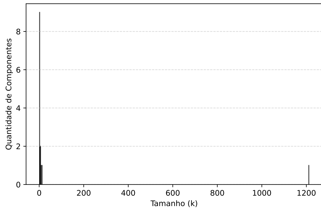
Grafo 1: Temas
