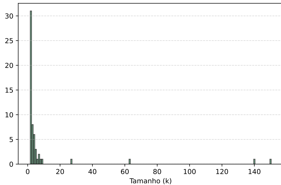
Grafo 2: Atributos
