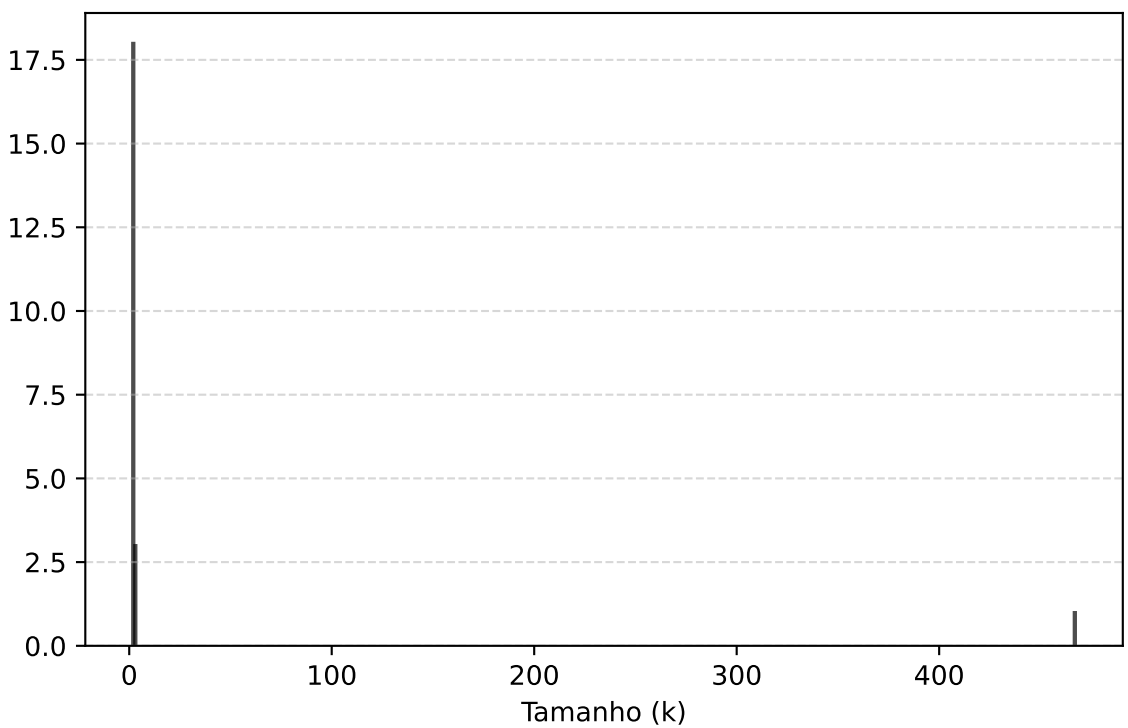
Grafo 3: Semântico
