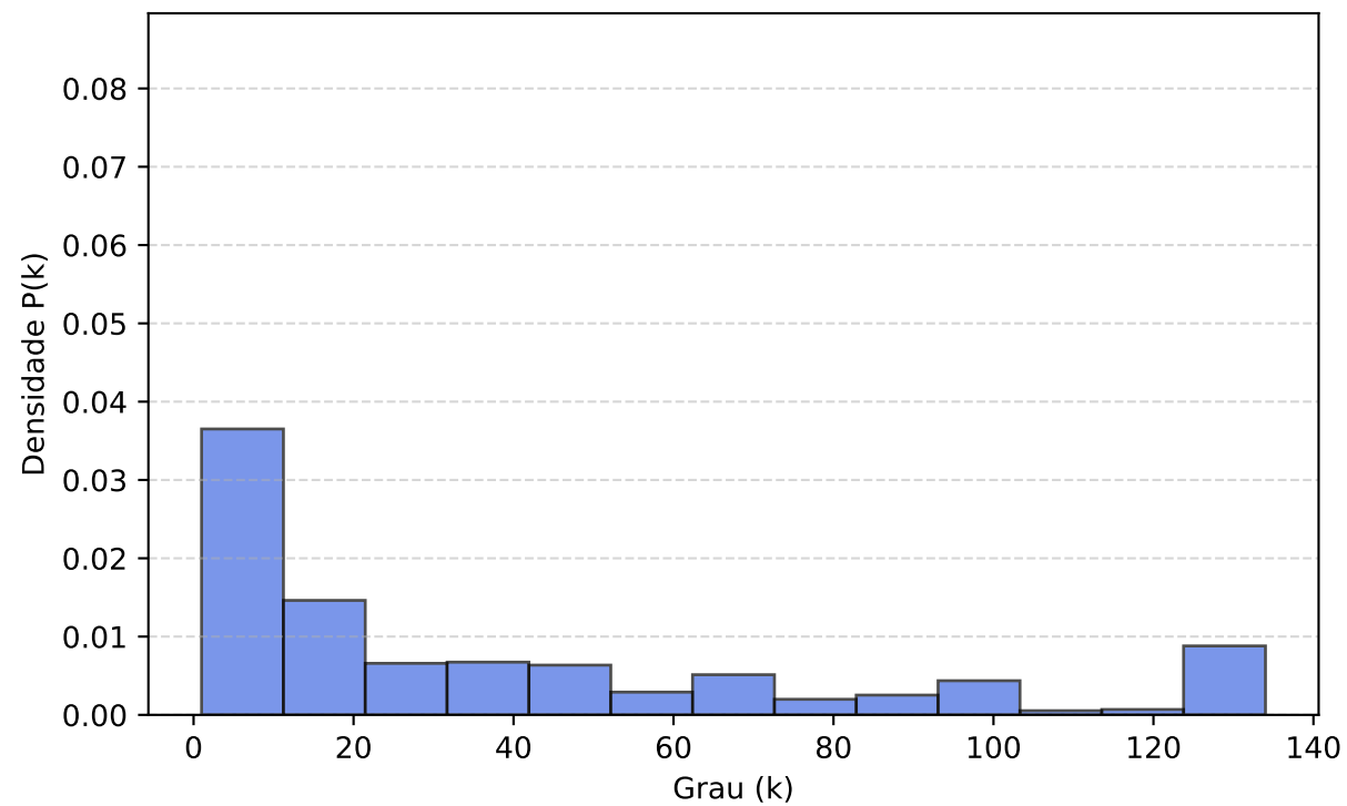
Grafo 1: Temas
