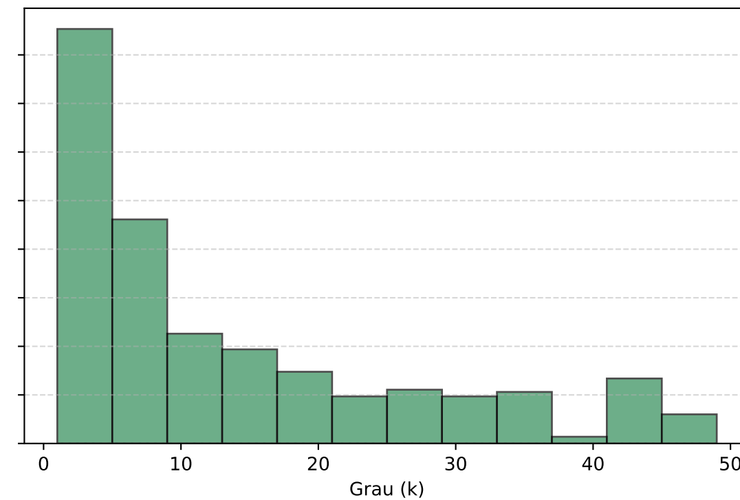
Grafo 2: Atributos
