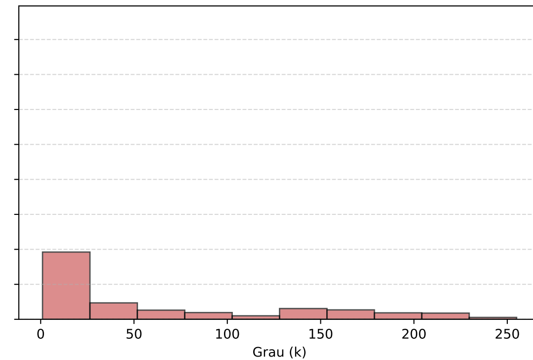
Grafo 3: Semântico
