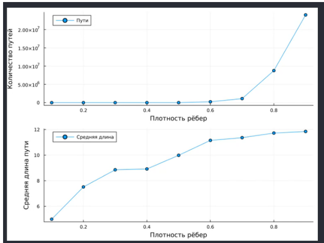
Рисунок 11: Полученный график - результат выполнения parameter_sweep.jl
