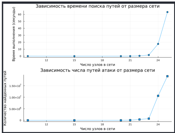
Рисунок 9: Сохранённый файл - результат выполнения convergence.jl
