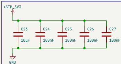
DECOUPLING CAPS
