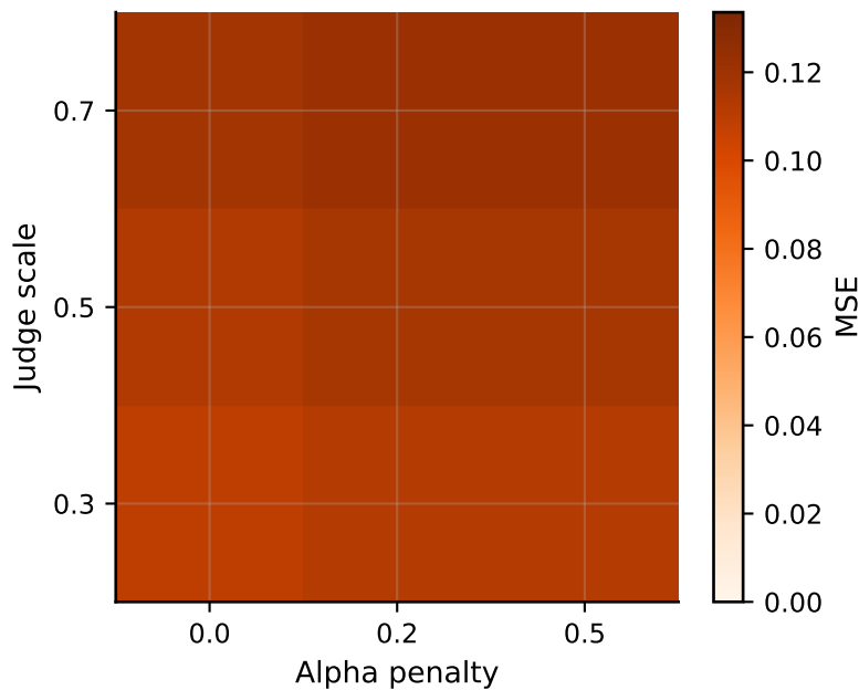
(b) Rank error (MSE)
