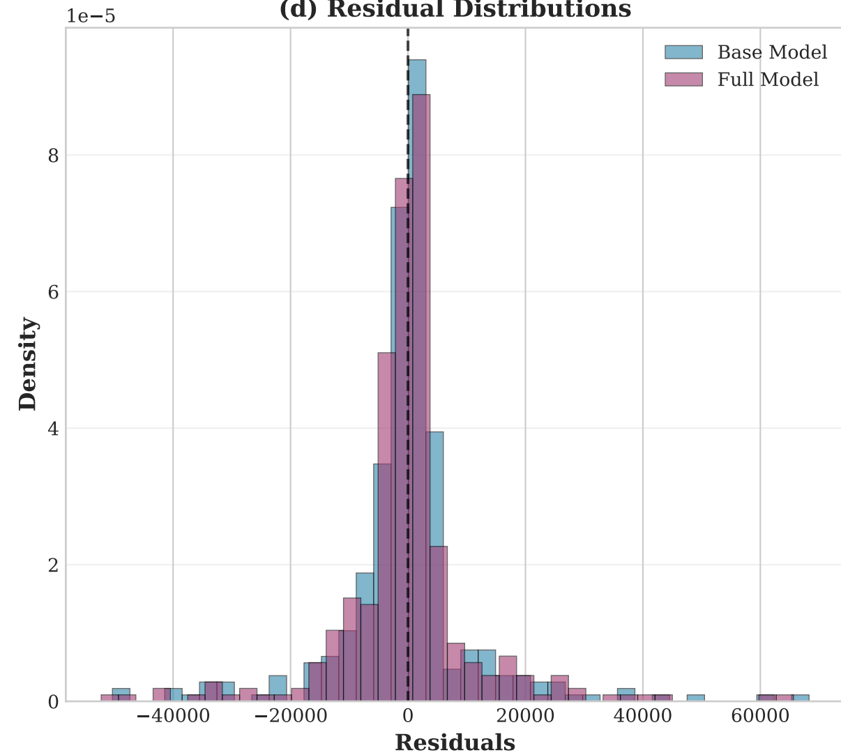
(d) Residual Distributions
