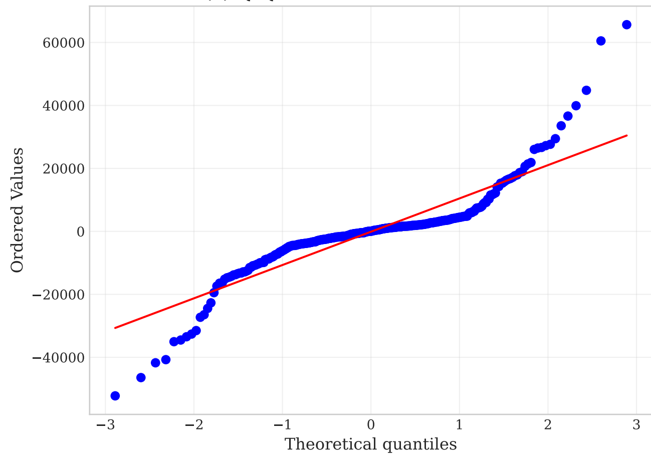
(d) Q-Q Plot: Full Model Residuals
