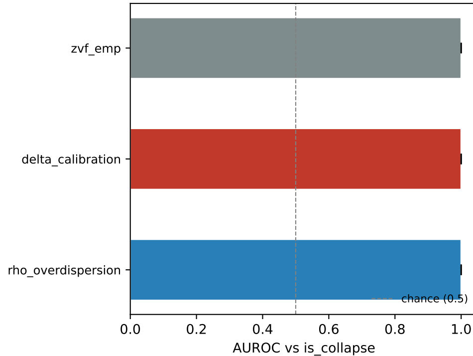
(a) Discrimination (AUROC)
