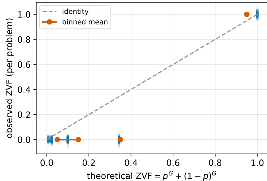
Frontier Qwen3-8B/GSM8K (n=600) obs-vs-theory r=0.93
