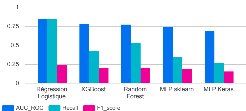
Comparaison des 5 modèles : AUC, Recall, F1
