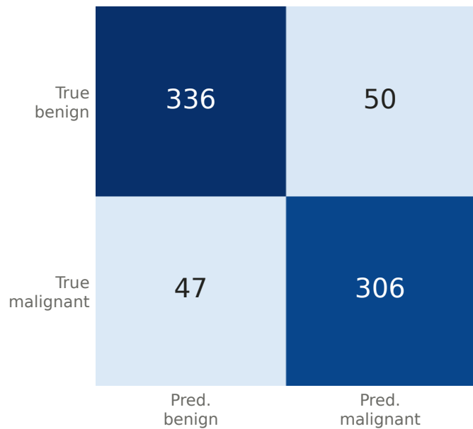
(d) Lesion-only + AttnMIL
