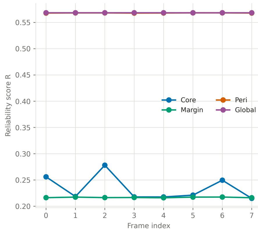
(d) Reliability across frames, real patient 2245 (DER-MIL; 8 valid frames)
