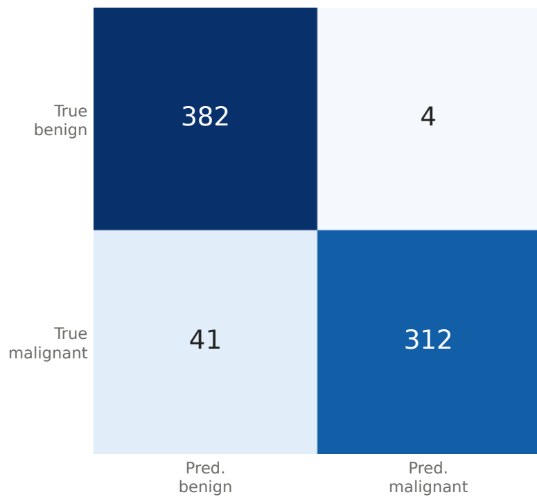
(d) RCAF
