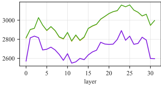
o_proj
