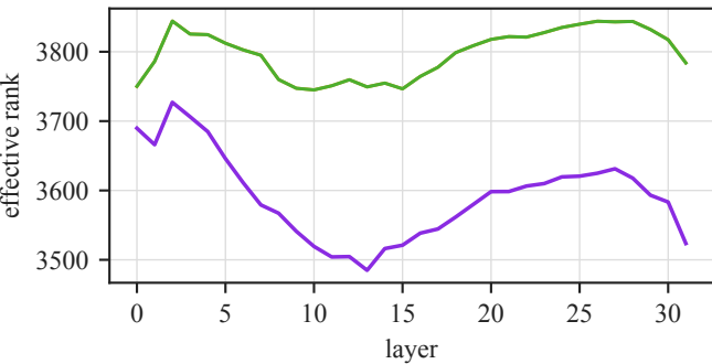
gate_proj
