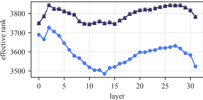
gate_proj
