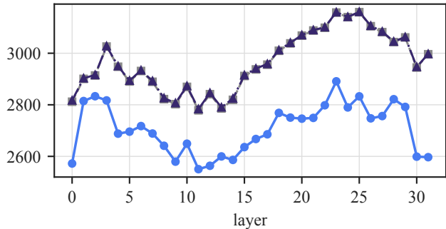
o_proj
