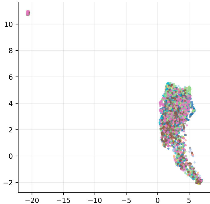
xlm-roberta-base UMAP
