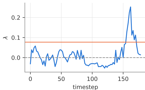
TurnOnSinkFaucet (demo 185)
