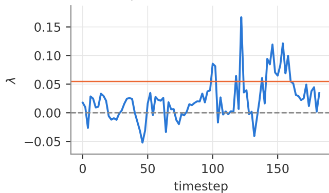
TurnOnSinkFaucet (demo 185)
