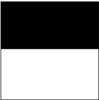
TDR: 1.0000
