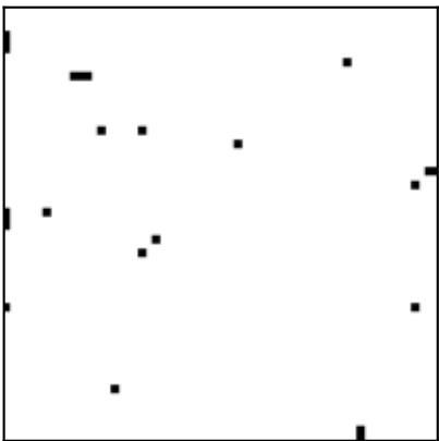
TDR: 0.9992
