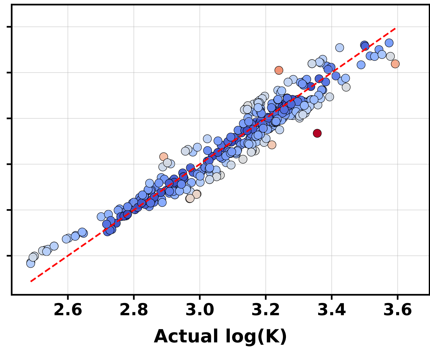
SVR
