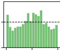
CSPX.L EWMA
