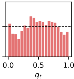
VUAG.L GJR(1,1,1)
