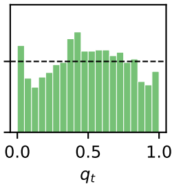
VUAG.L EWMA
