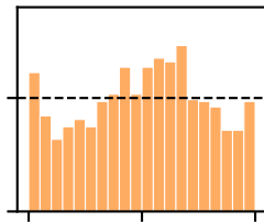
CSPX.L RiskMetrics
