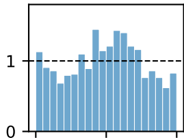
CSPX.L GARCH(1,1)
