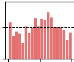
CSPX.L GJR(1,1,1)
