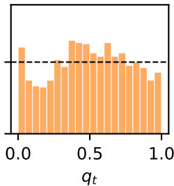
VUAG.L RiskMetrics
