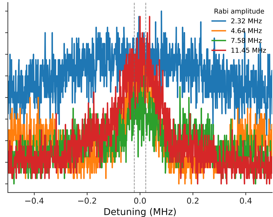
Lorentzian zoom
