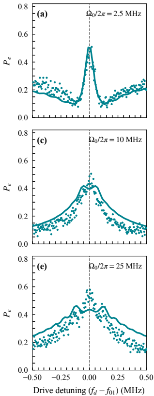
Root-Lorentzian
