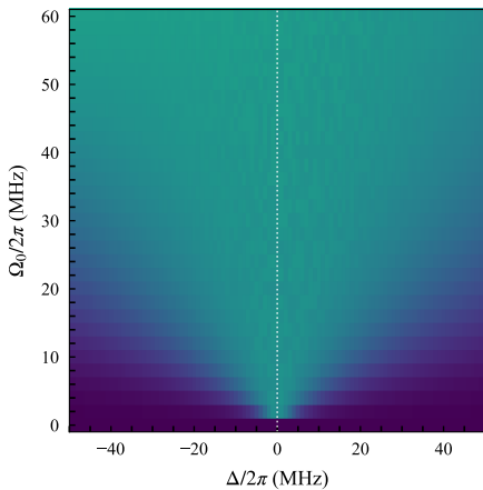
(d) Constant: 20 MHz zoom
