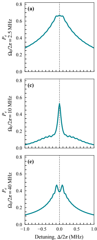
Root-Lorentzian
