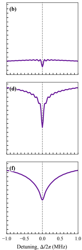
Echo-root-Lorentzian
