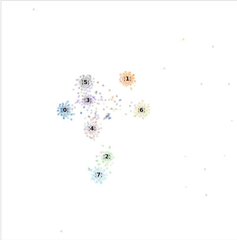
LAMP-Merge
