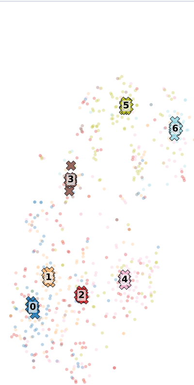
LAMP-Merge
