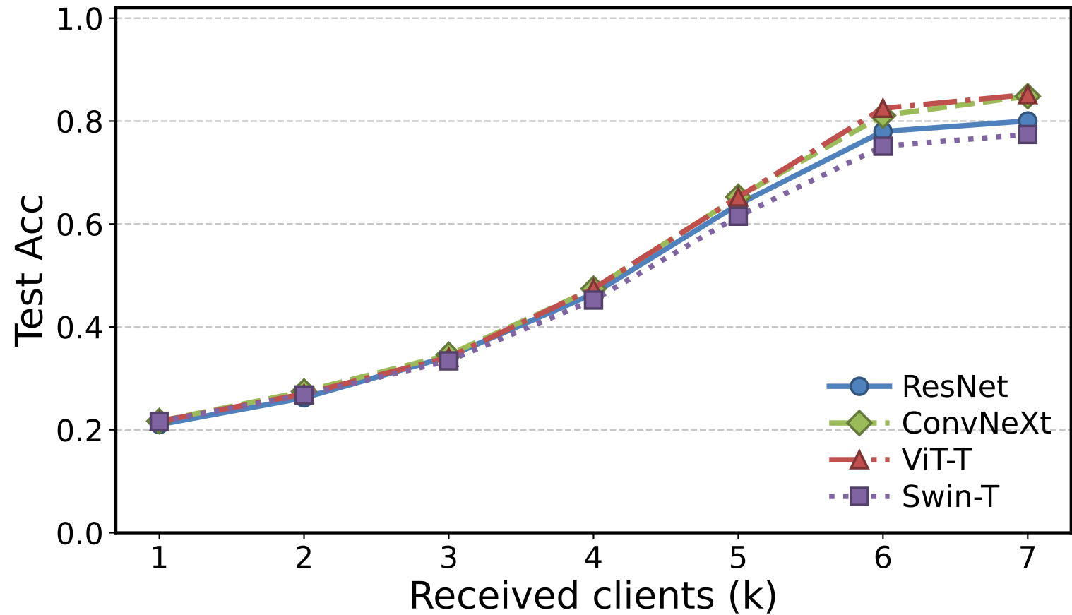
BloodMNIST: Acc
