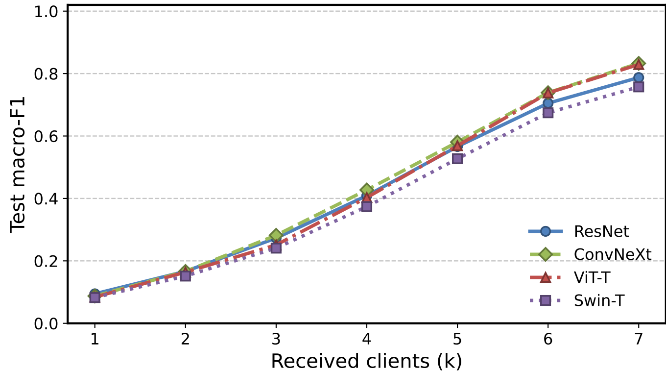
BloodMNIST: Macro-F1
