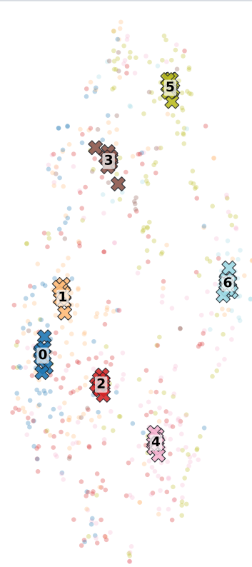
LAMP-Merge
