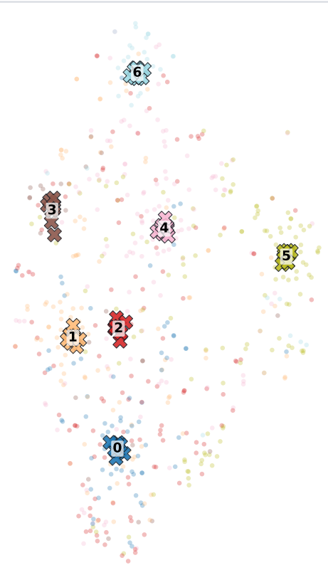
LAMP-Merge
