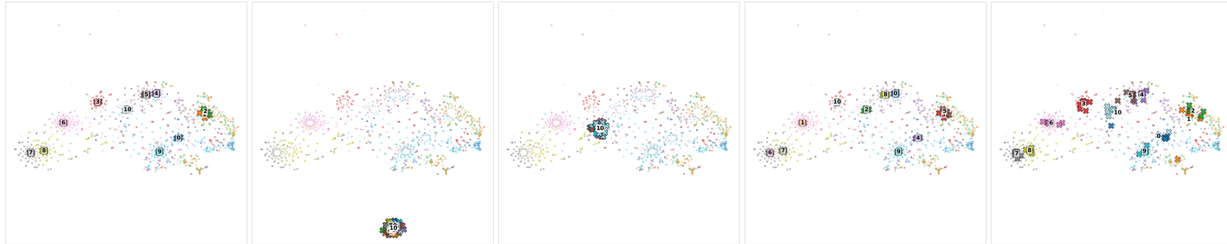
LAMP-Merge
