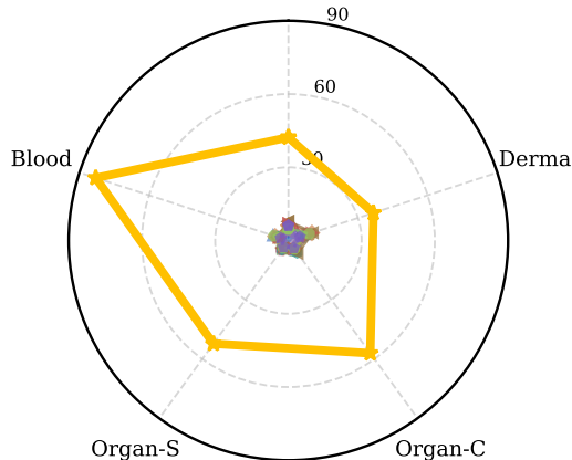
F1 Ultrasound
