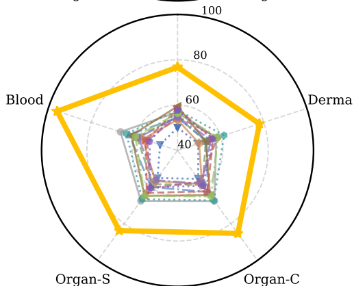
AUC Ultrasound
