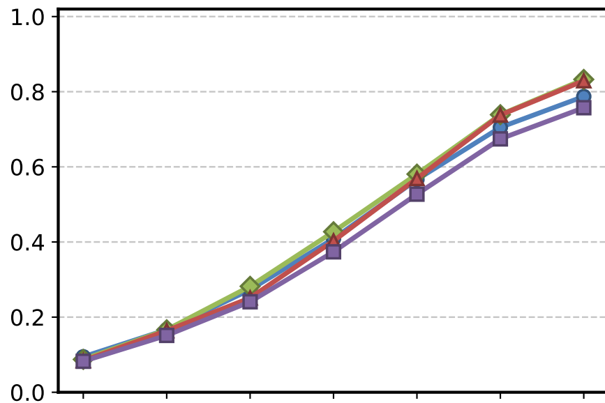
BloodMNIST
