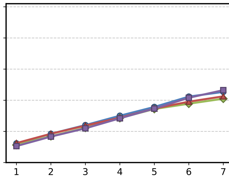
UltrasoundMNIST
