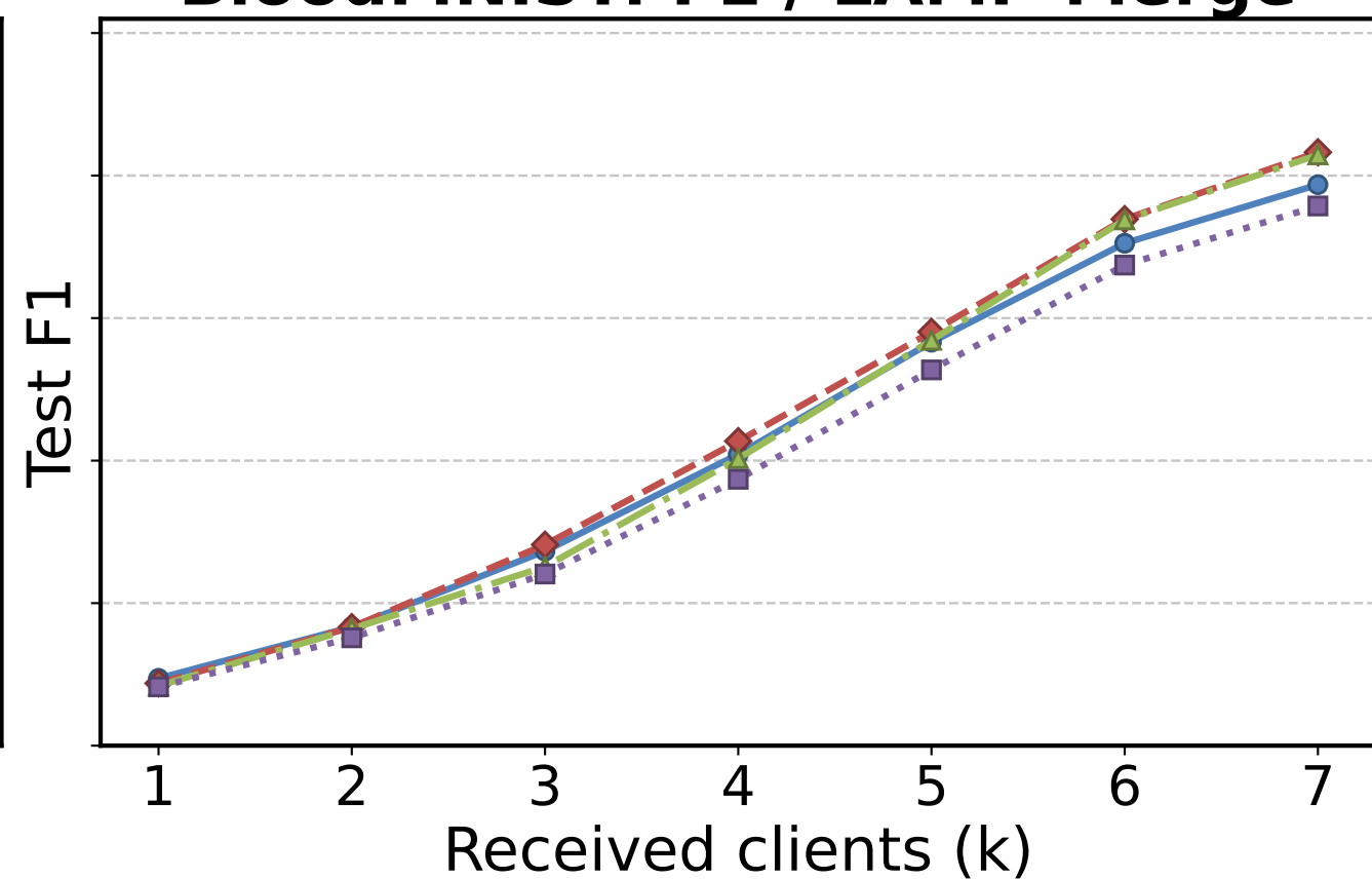
BloodMNIST: F1 / LAMP-Merge
