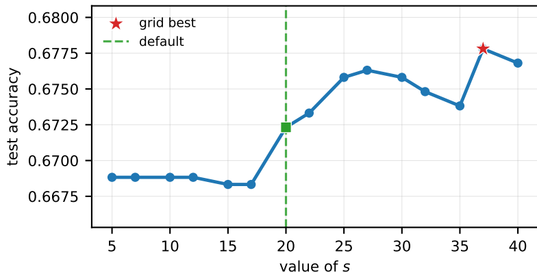
M1: s
