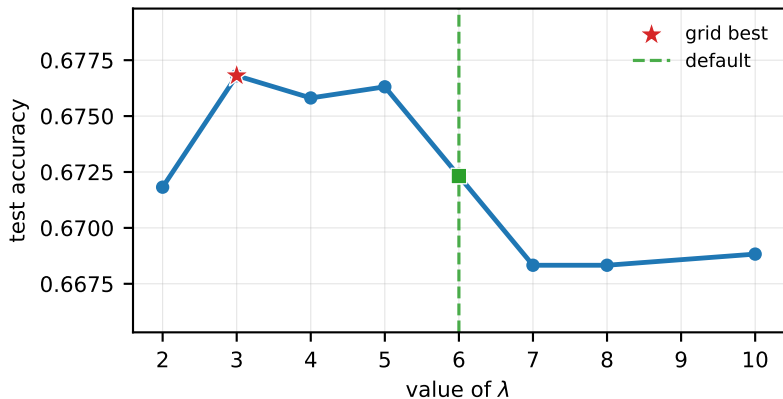
M2: \lambda
