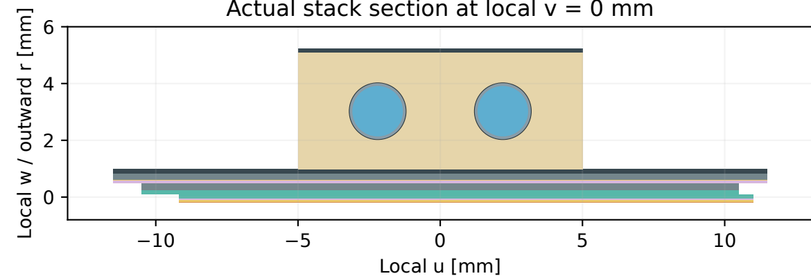
Actual stack section at local v = 0 mm
